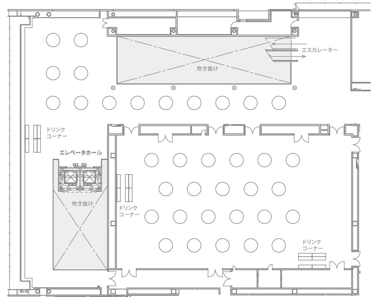
円卓使用(36卓、700名)
