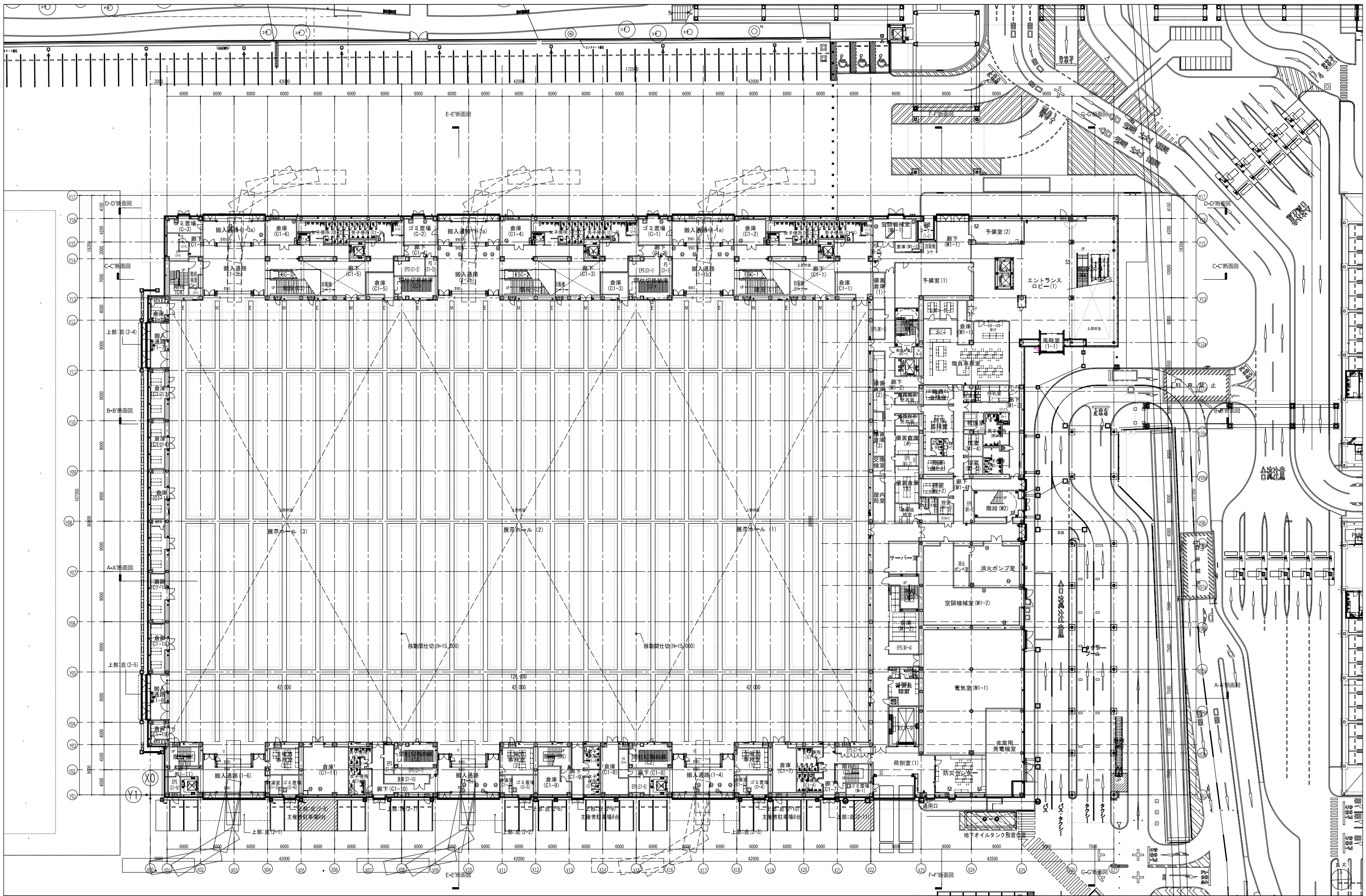
1階平面図 縮尺: A1 1:300 A3 1:600
